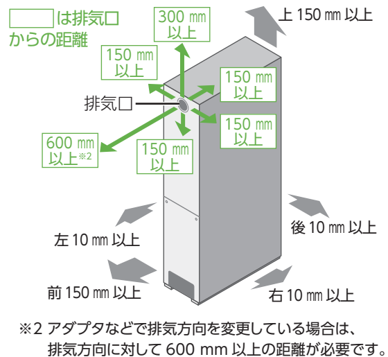
貯湯ユニット
